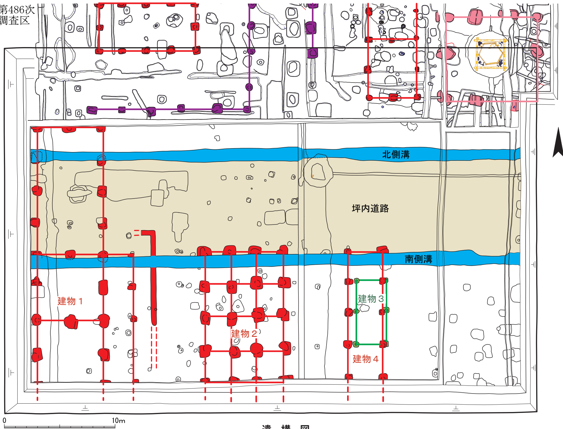
遺構図
